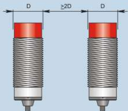
Montaggio affiancato
