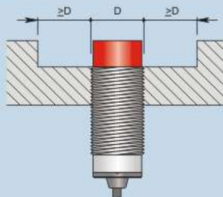
Montaggio sporgente
